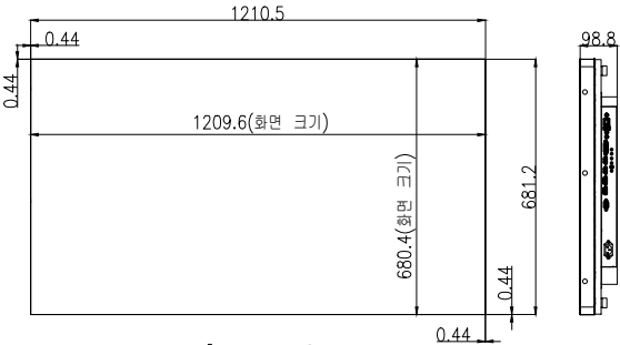
[55"멀티모니터]
