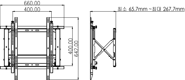
[팝업 브라켓]
